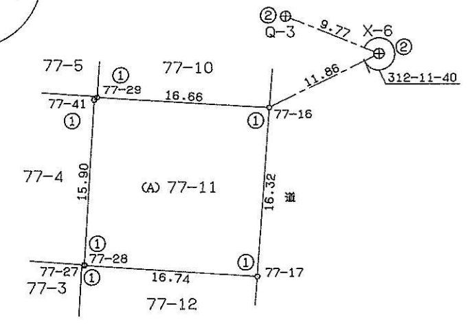
拡大図 S=1:50
